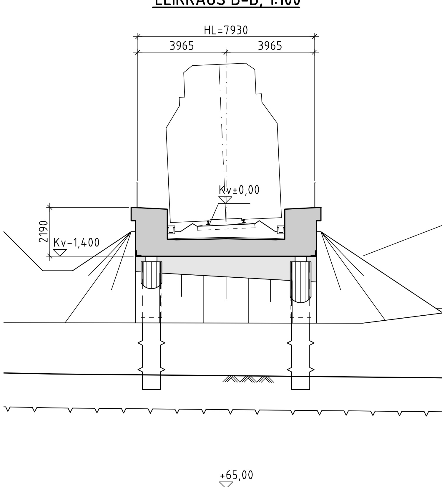
LEIKKAUS B-B, 1:100
