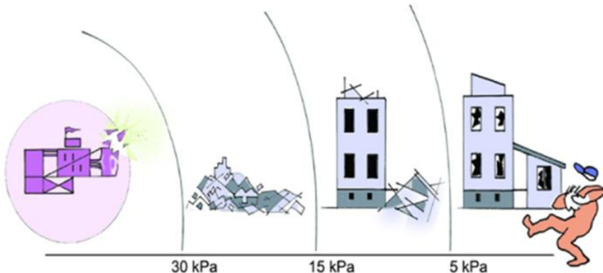
Kuva 5: Paineaallon vaikutuksia (Lähde; Tukes-opas Tuotantolaisten sijoittaminen, 2025, piirroks: Pirkko-Liisa Toppinen.)
