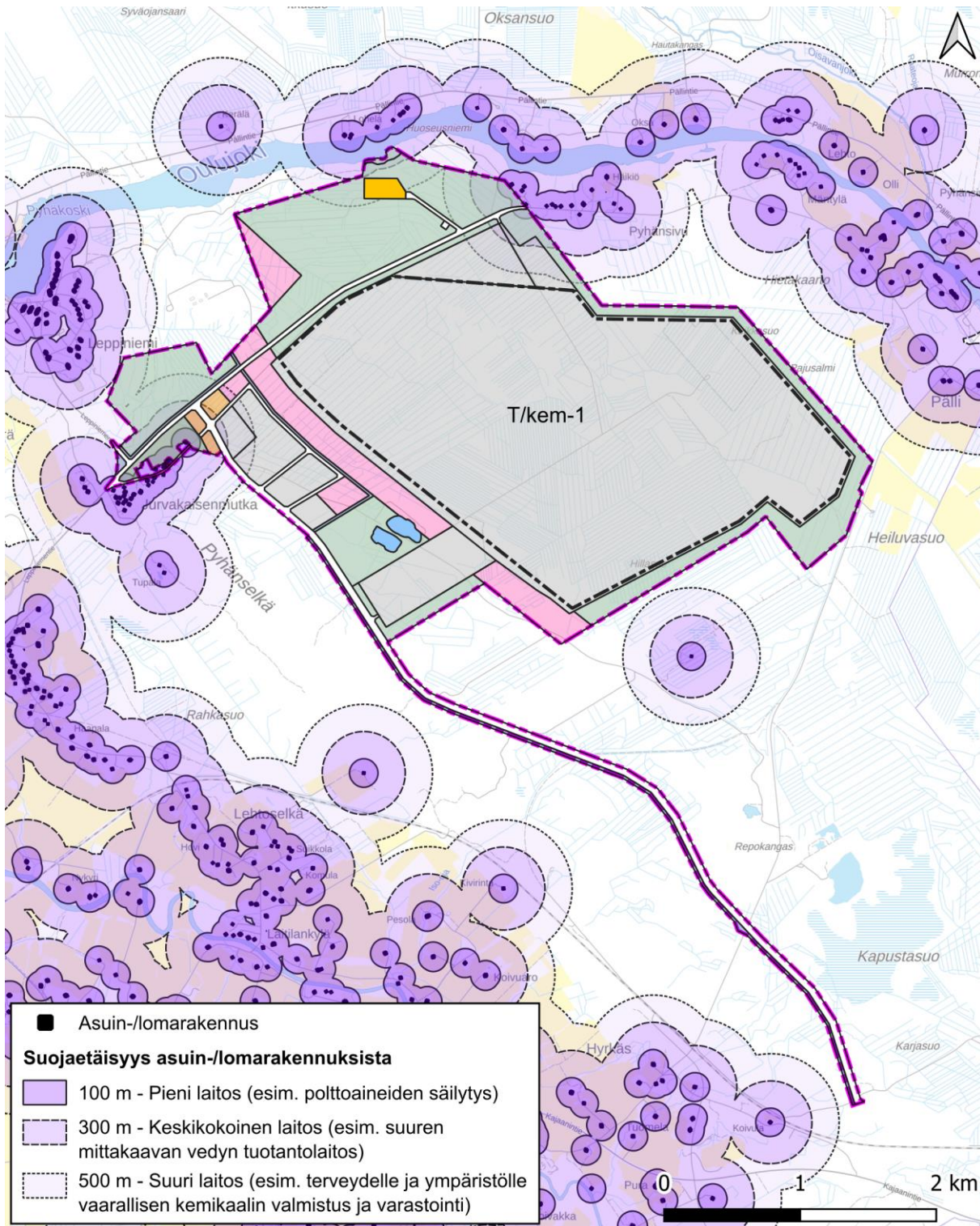
Kuva 6: Alueen asuin- ja lomarakennusten ympärille piirretyt laitoskohtaiset suojaetäisyydet (rakennustiedot: MML 2025). Asemakaavaehdotuksen mukainen T/kem-1-alueen rakennusala on esitetty mustalla paksulla pistekatkoviivalla.
