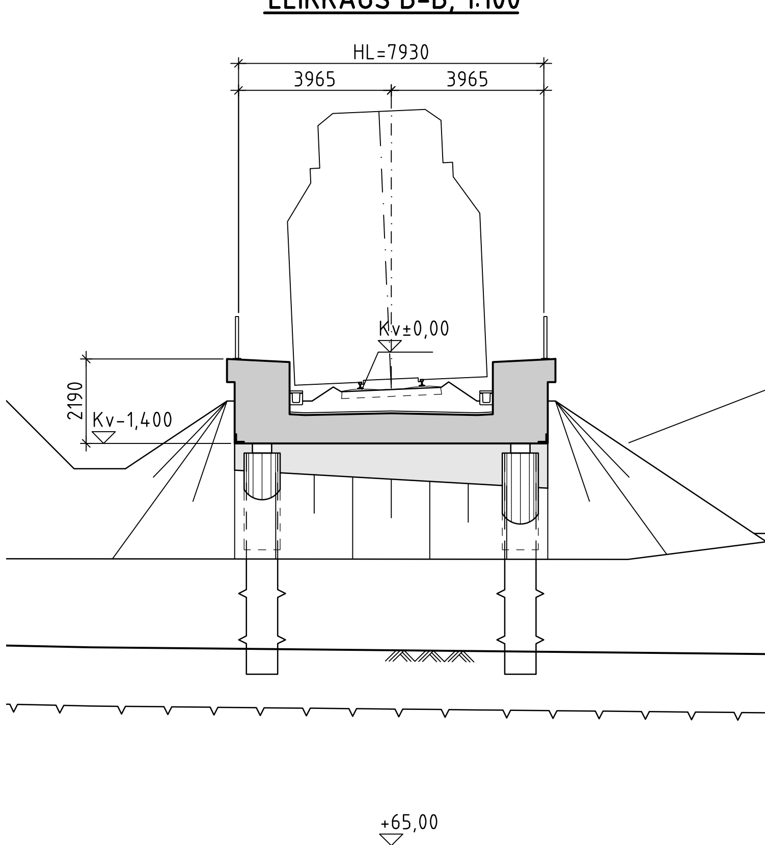
LEIKKAUS B-B, 1:100
