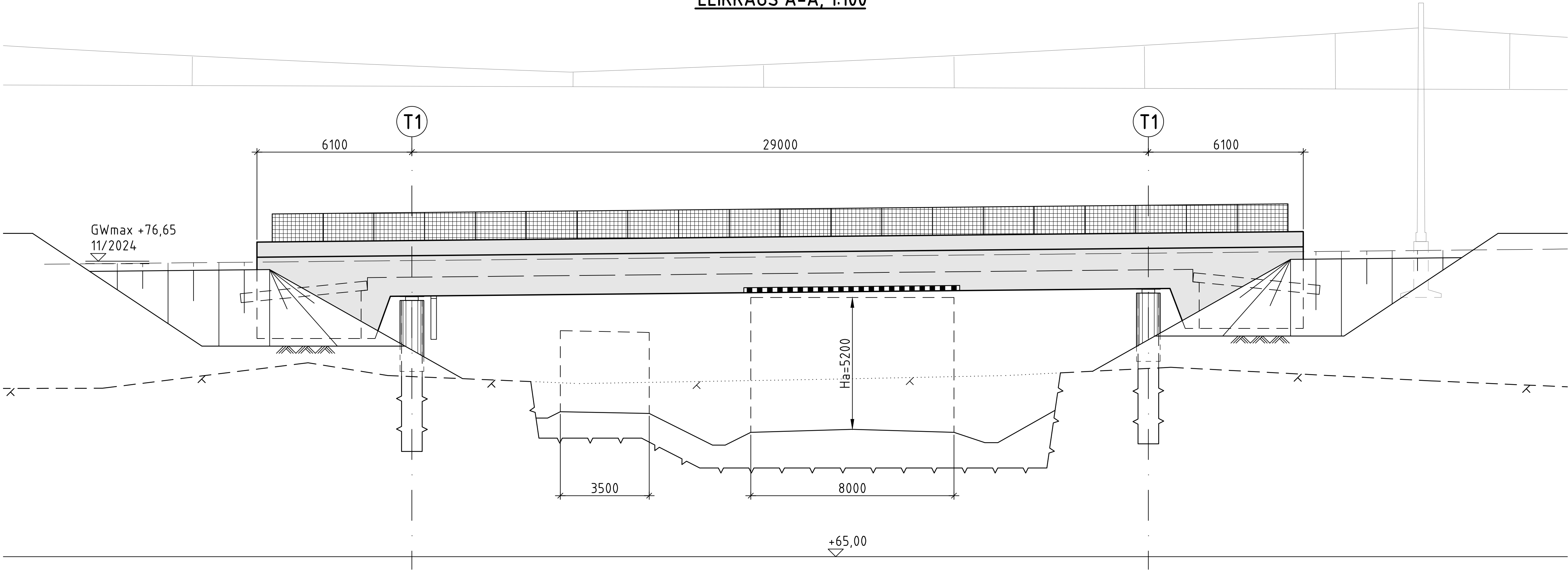
LEIKKAUS A-A, 1:100
