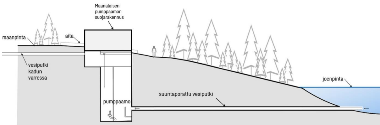
Kuva 84. Periaatteellinen leikkauskuvio teollisuuden mahdollisesti tarvitseman prosessiveden pumppaamosta. Kuva esittää teoreettisesti, miten vesistön pohjasta otettavan prosessiveden pumput sijaitsevat syvällä maan sisässä ja pumppaamokaivantoa peittää tekninen rakennus sekä sen, että teknisen huollon alue aidataan. Suuntaporaus tarkoittaa, että vesistön ja pumppaamon väliseen ympäristöön ei tule näkyviä rakenteita.
